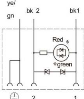
抑制二极管带过压保护+红/绿灯 12V
