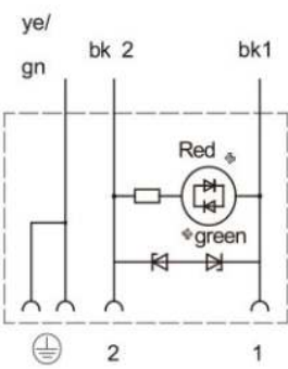
抑制二极管带过压保护+红/绿灯
