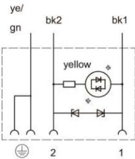
抑制二极管带过压保护 + 黄灯
