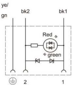
抑制二极管带过压保护+红/绿灯
