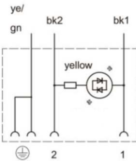
无抑制二极管带过压保护 + 黄灯
