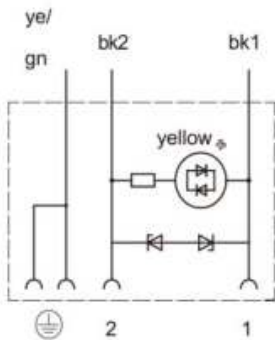
抑制二极管带过压保护+黄灯
