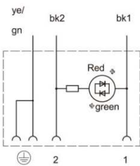
无抑制二极管带过压保护+红/绿灯
