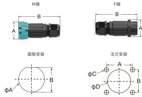
尺寸图 Dimension drawing
